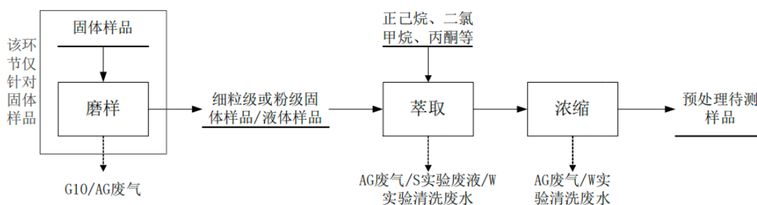
图3-3 制样及样品前处理实验流程及产物节点示意图
